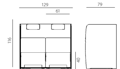
RUBICO LOUNGE 102
